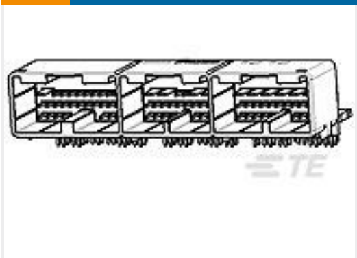
TE 产品编号1318751-4 025/090 80P CAP HSG ASSY AU RN
