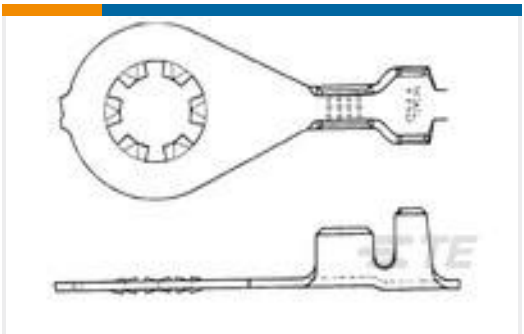
TE 产品编号626283-4 TERMINAL
