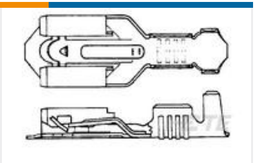
TE 产品编号881598-2 RECEPTACULO 50 MM
