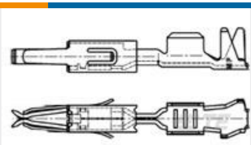
TE 产品编号964275-2 MT2 A REC 1.6 Contact SWS Sn (LP)
