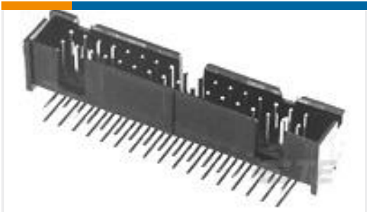
TE 产品编号103310-3 016 LOPRO HDR RA 15DP
