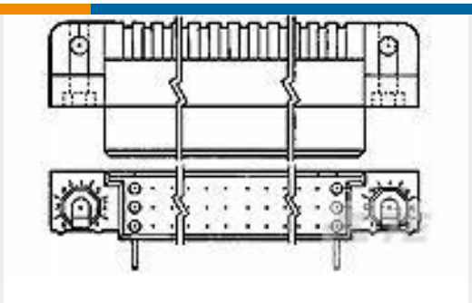
TE 产品编号1-532431-3 HDI RECP ASSY 3 ROW 240 POS
