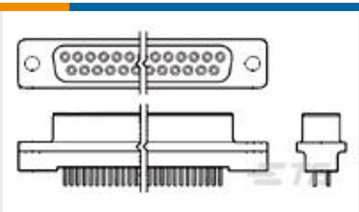
TE 产品编号5745078-5 HD-20 RCPT 25P VERT FFSCRLK
