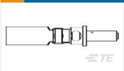
TE 产品编号622649-000 D-600-0018
