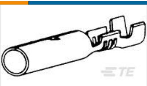
TE 产品编号42531-1 180 SHPL REC 20-16 016BR
