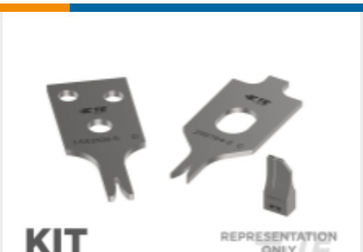
TE 产品编号7-2836562-7 OC-102F116O-CRIMPTOOLINGKIT
