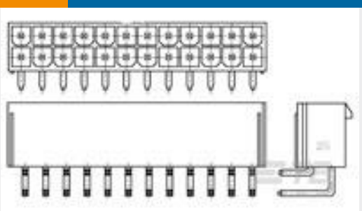
TE 产品编号2-1586042-2 22P VAL-U-LOK R/A HDR V0
