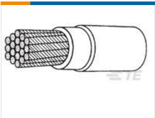
TE 产品编号828923-000 82A0813-8-9
