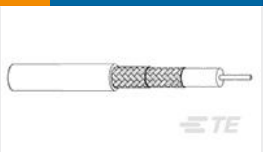
TE 产品编号420106-002 5020A3311-0
