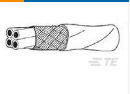
TE 产品编号3180673002 55A1841-22-2/4/5/6-9
