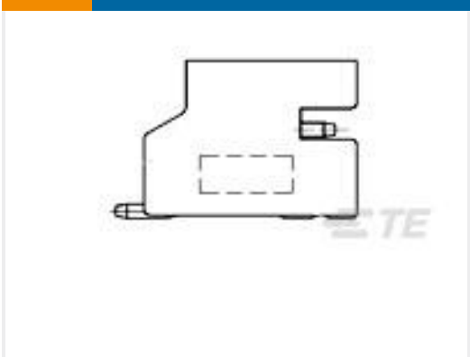
TE 产品编号1-1775469-3 HPI CONN., 2.0MM, R/A, SMT, 13P, 80U"
