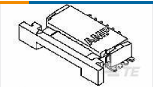
TE 产品编号1-84952-4 1MM FPC HORZ.BTTM CONT.ASS.14P
