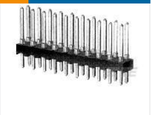
TE 产品编号2-87227-2 44 MODII HDR DRST UNSHRD .100
