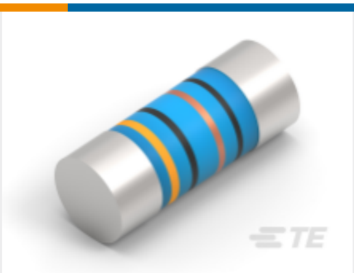
TE 产品编号1-2176316-7 MELF SMA_A 2K2 0.1% 15PPM 0207 1W
