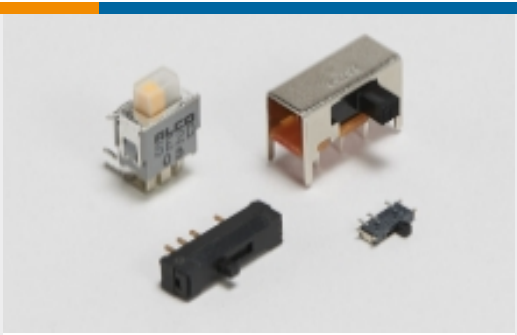
滑动开关(63)
