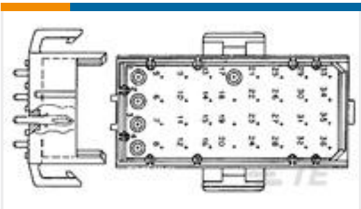
TE 产品编号2-640504-4 20P MR HDR ASSY VO RED LF
