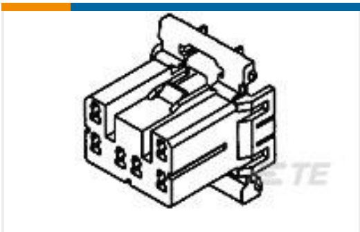
TE 产品编号173853-1 070 MULTILOCK PLUG 18P
