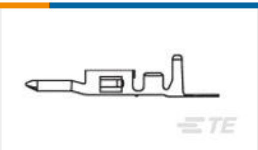
TE 产品编号1586054-1 VAL-U-LOK PIN BR SN 16AWG
