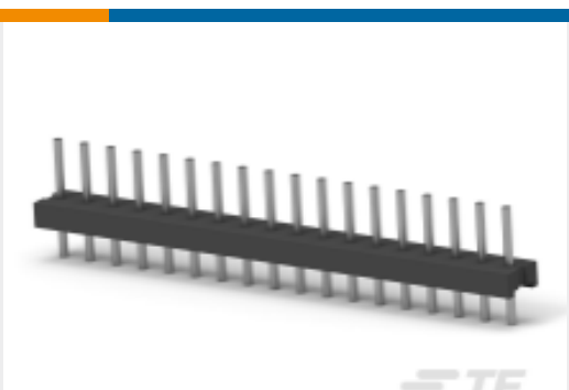
TE 产品编号 1-644750-8 18P MTA156 HDR ASSY STR RND SN
