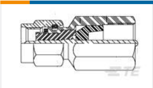
TE 产品编号1-1337558-0 FME Str Plg-SMAP Adp Nickel Pltd
