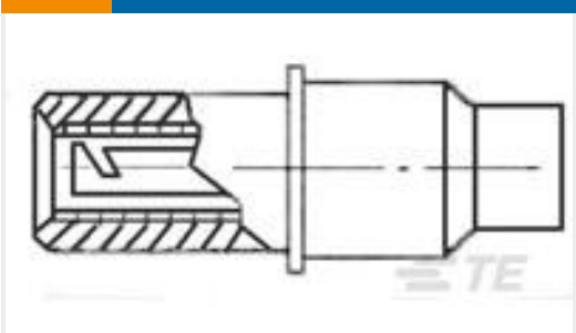
TE 产品编号147424-000 D-602-1111
