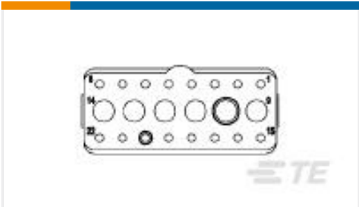
TE 产品编号1738149-1 Insert Asy,Socket, GPRBE22SA
