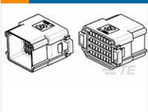
TE 产品编号1981556-1 ME M D1100 24P-R TAB HSG ASSY
