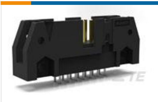
TE 产品编号1-5102153-2 A/L UNIV HDR 64P VERT
