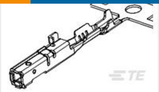
TE 产品编号1827483-2 0.64 III RCPT NON SEALED AU (SS)
