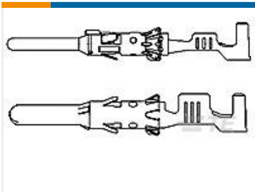
TE 产品编号1703018-1 DIA 1.5MM CONTACT PIN,LP
