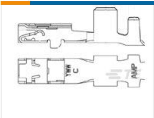
TE 产品编号1326030-1 2.8MM RECP,UNSEAL,22AWG
