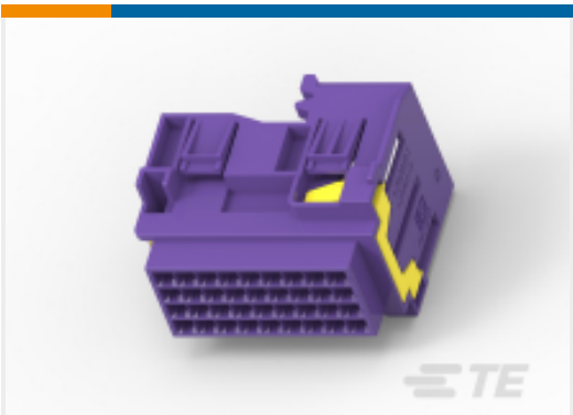
TE 产品编号1-2112891-2 36POS, TAB 1.5x0.6, TAB HSG, ASSY
