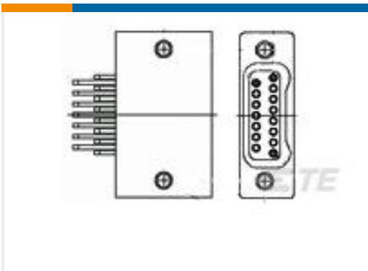
TE 产品编号2-1589483-7 STL065L2HN = SMT CONN
