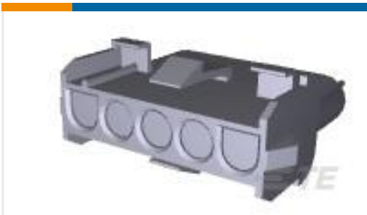
TE 产品编号1-480764-0 05P UMNL CAP HSG NATL
