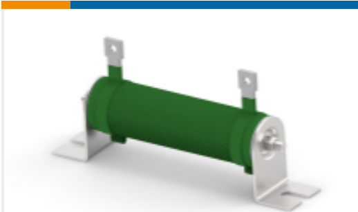
TE 产品编号1879447-3 线绕电阻器：矿物，2.5 Kw
