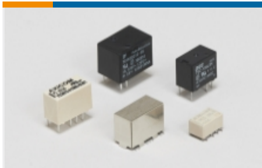
信号继电器(33)
