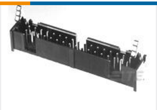
TE 产品编号3-1761606-6 IDC LOW PRO HDR 60P VERT LG LA
