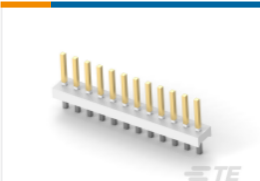
TE 产品编号 4-644763-2 12P MTA156 HDR ASSY STR AU LF
