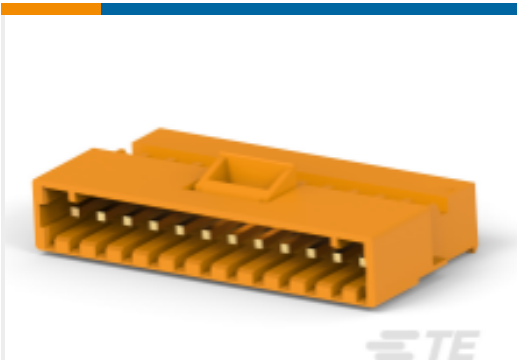
TE 产品编号 4-647476-2 12P MTA156 PSTD CONN 18AWG LF
