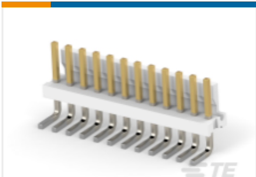
TE 产品编号 4-644768-2 12P MTA156 HDR ASSY F/L SQ LF
