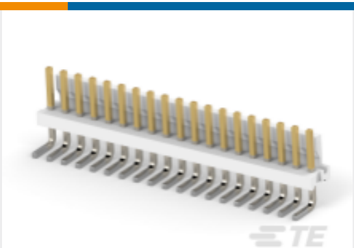
TE 产品编号 4-644768-9 19P MTA156 HDR ASSY F/L SQ LF
