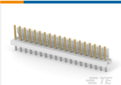
TE 产品编号 4-644767-9 19P MTA156 HDR ASSY FL ST LF
