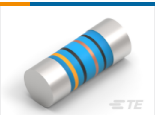
TE 产品编号1-2176314-3 MELF SMA_A 1K0 0.1% 15PPM 0102 0.3W
