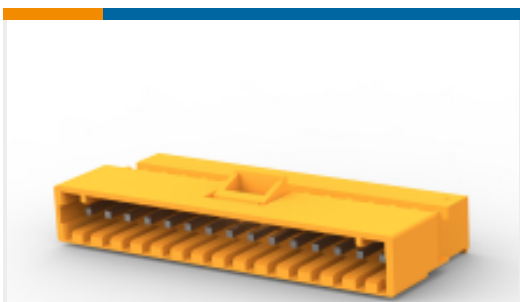
TE 产品编号 4-641435-5 15P MTA156 CONN ASSY ORNG
