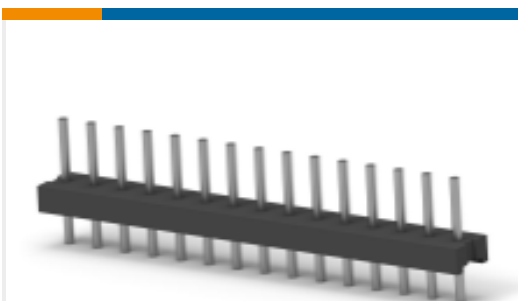
TE 产品编号 1-644750-5 15P MTA156 HDR ASSY STR RND SN
