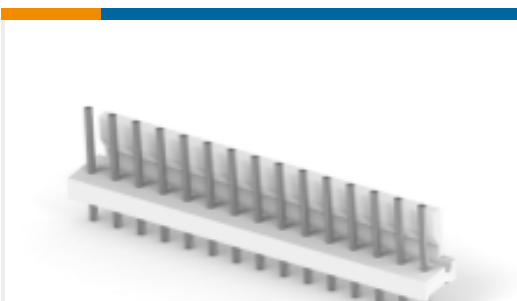
TE 产品编号 1-644753-5 15P MTA156 HDR ASSY RN STR F/L
