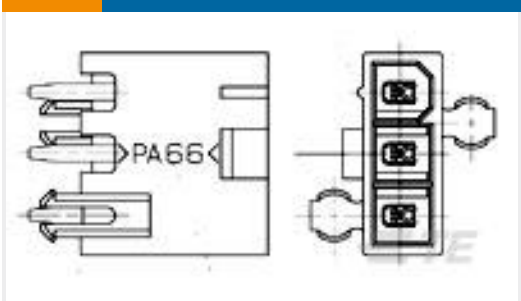
TE 产品编号2029167-5 5P VAL-U-LOK SR HDR SN V0 WODH
