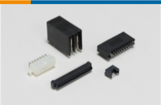
PCB 连接器键控(6)
