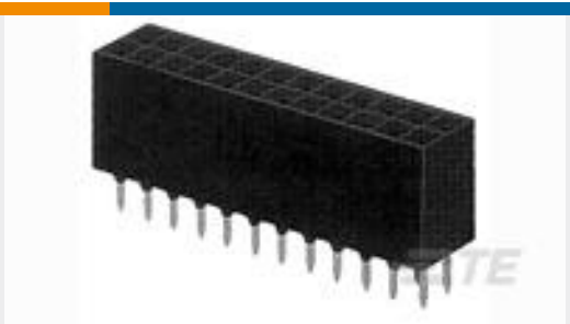
TE 产品编号 6-534236-5 30 MODII VRT DR CE 100/120 NO KINK
