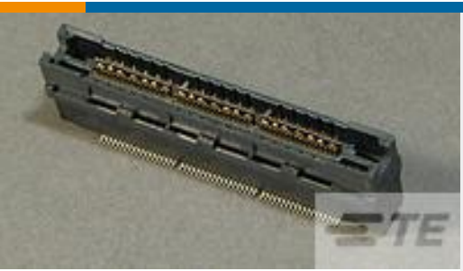
TE 产品编号 767145-3 MICTOR .355 EXTENDED HEIGHT RECEPTACLE,
