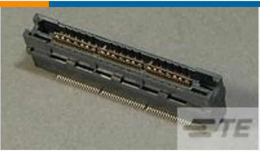
TE 产品编号 767130-3 MICT,RCPT,114,ASY,GOLD,EXTD
