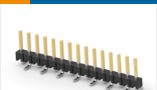
TE 产品编号 1-147306-3 15 MTE HDR HSG SR LATCH .100
