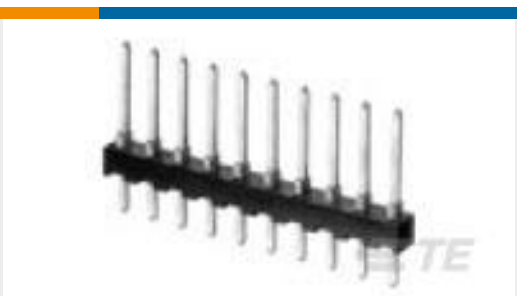
TE 产品编号 1-87224-5 15 MODII HDR SRST UNSHRD .100
