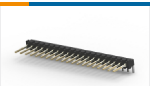
TE 产品编号 1-2267063-5 15 MODII HDR SRRA UNSHRD .100
