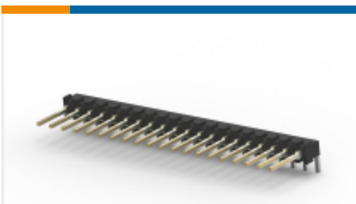
TE 产品编号 6-2267063-5 15 MODII HDR SRRA UNSHRD .100
