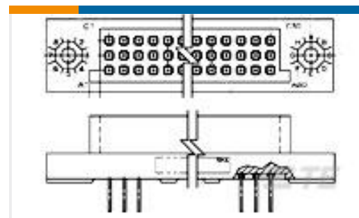
TE 产品编号1-447208-5 3 ROW BOX RECP 240 POS 100 C/L
