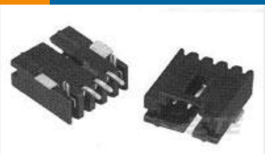
TE 产品编号 147323-4 05 MTE HDR SRRA SMT.100CL
