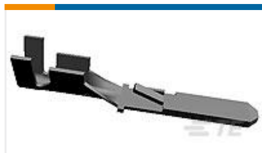
TE 产品编号160887-4 FF 110 TAB 0.5-1.0MM2 PTPPB
