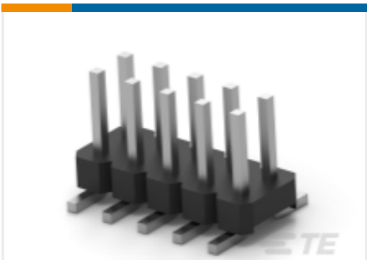
TE 产品编号2842144-4 8P,2MM,BRK HDR,DRVT,SMD,0.76AU, TR W/CAP
