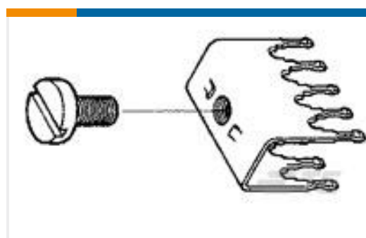
TE 产品编号 1-5055558-1 10 PWR TAP CONT PLTD MTR .100
