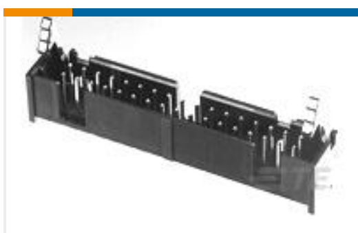
TE 产品编号 1761608-6 IDC LOW PRO HDR 16P VERT SHT LAT BLK
