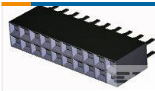
TE 产品编号 6-534206-0 20 MODII VRT DR CE 100/115
