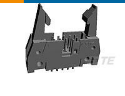
TE 产品编号1-499160-0 050 UNIV HDR SP 4S 30DP STD L2
